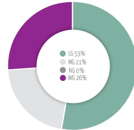
Typen 1975:
