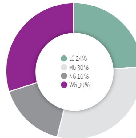
Typen 1986:
